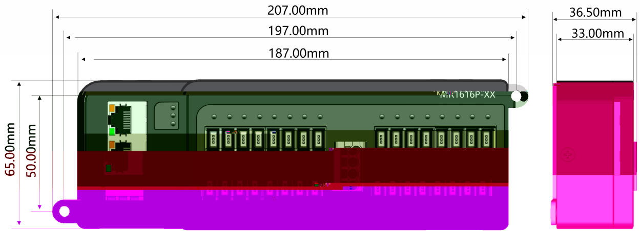
4 1--207 *65 W/H mm
